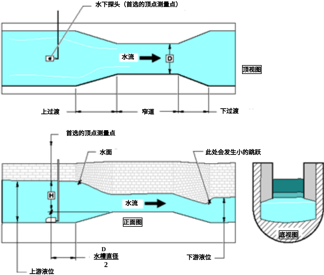
图 53 Leopold-Lagco 型水槽
